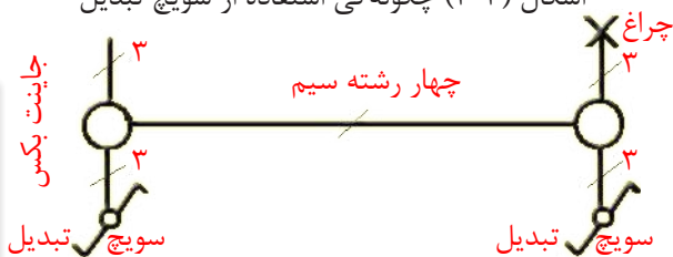
اشکال (۳-۳) چگونه گی استفاده از سوئیچ تبدیل
